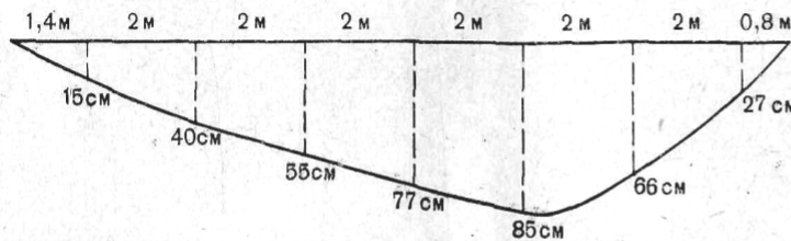
Рис. Поперечный профиль реки.
